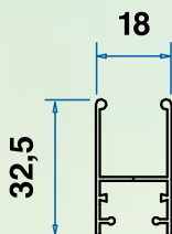
Guida alta due vie
