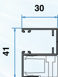
Guida 30x41
