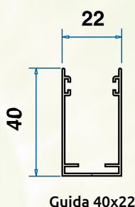
Guida 40x22
