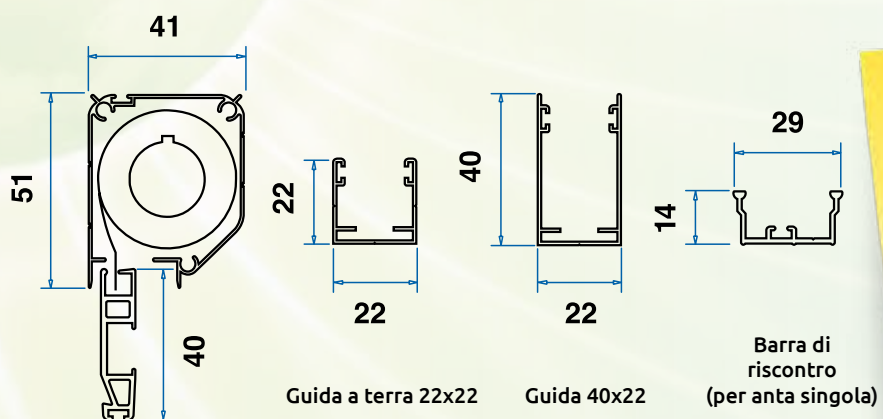
Cassonetto con tubo, rete e barra maniglia
