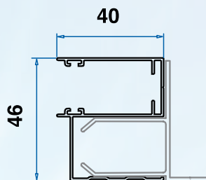
Guida 40x46
