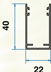
Guida 40x22
