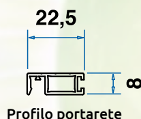
Profilo portarete
