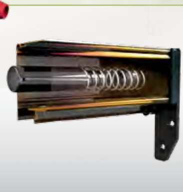
Freno Viscodinamico
