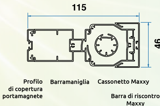
Barra di riscontro Maxxy
