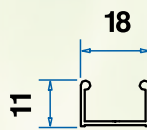
Guida a terra due vie
