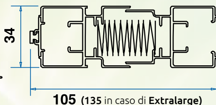
Barra di riscontro **
