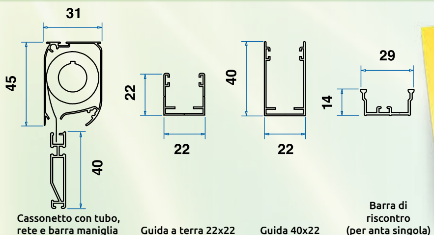
Guida a terra 22x22
