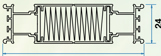
Profilo portarete
