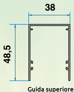
Guida superiore
